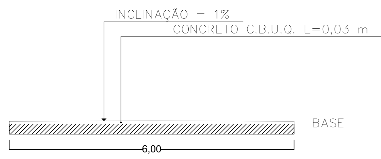
CORTE A-A
