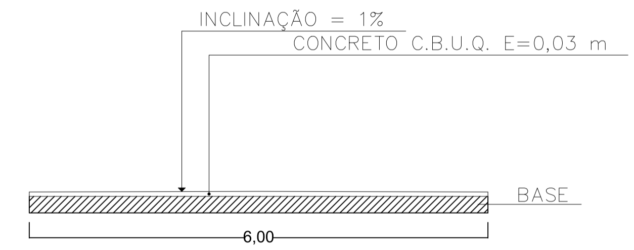
CORTE A-A
