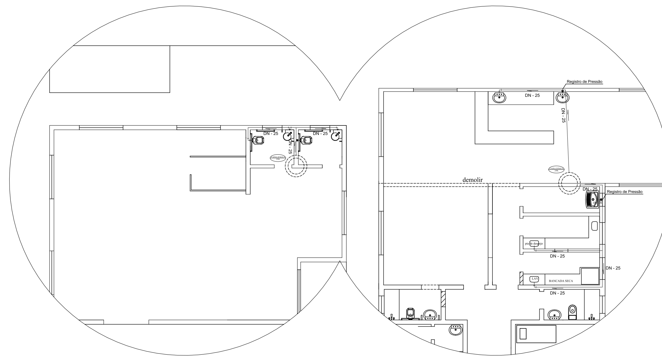
HIDRÁULICO PAV. TÉRREO esc. 1: 100
