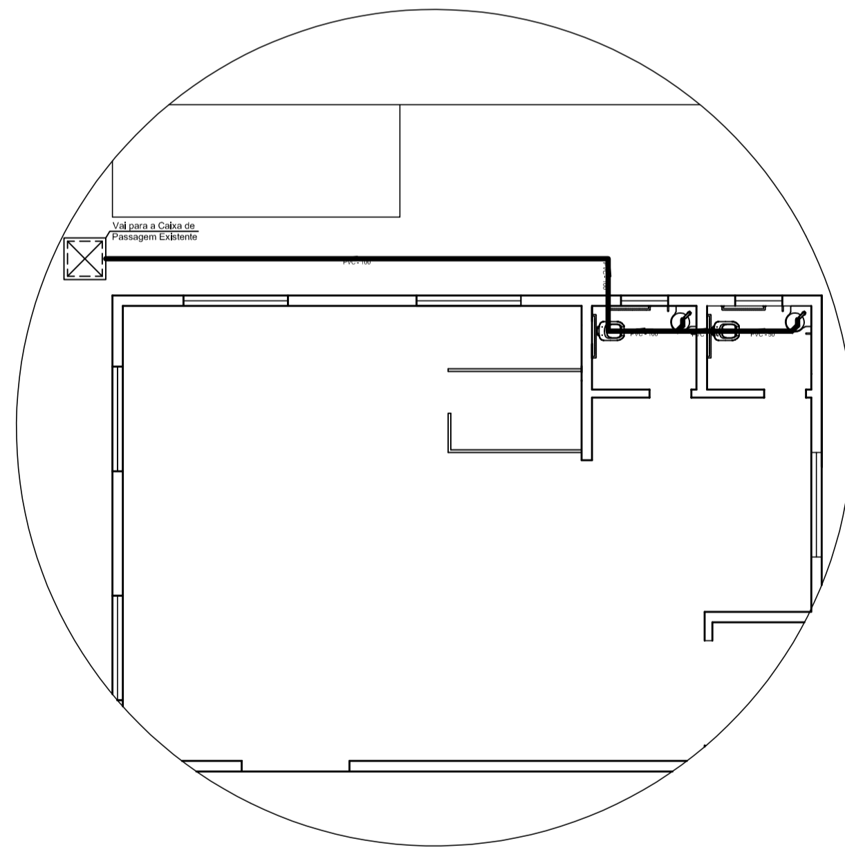
ESGOTO PAV. TÉRREO esc. 1 : 100
