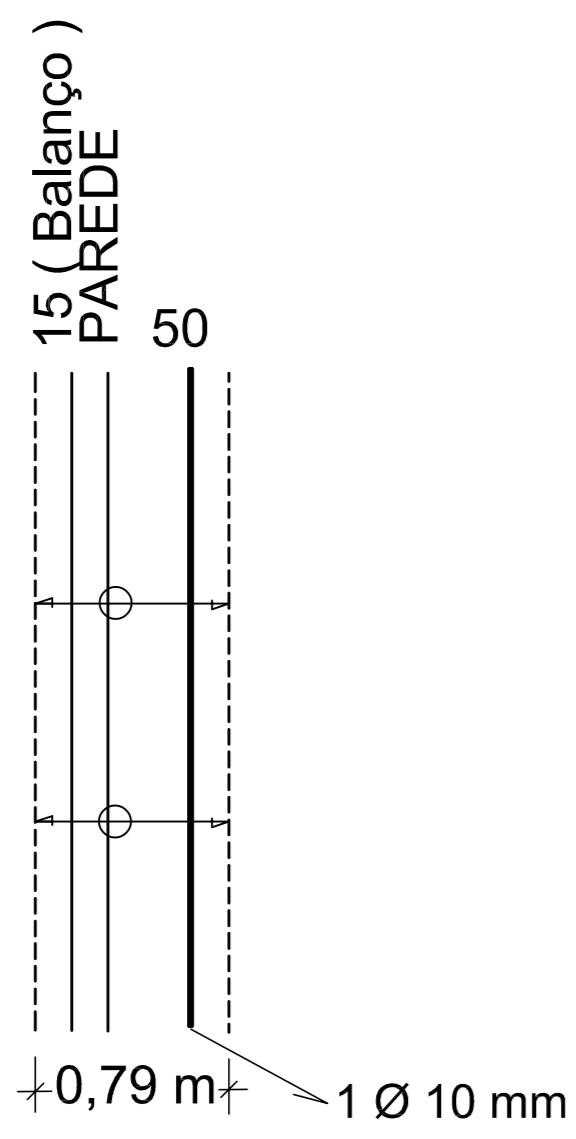
DETALHE BALANÇO LAJE
