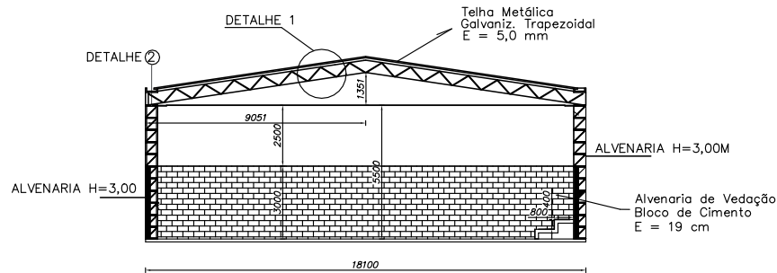
VISTA EM CORTE AA esc. 1:100
