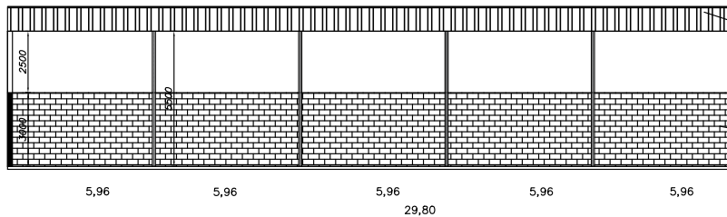
VISTA EM CORTE BB esc. 1:100
